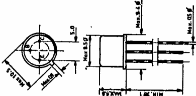
TO-5
