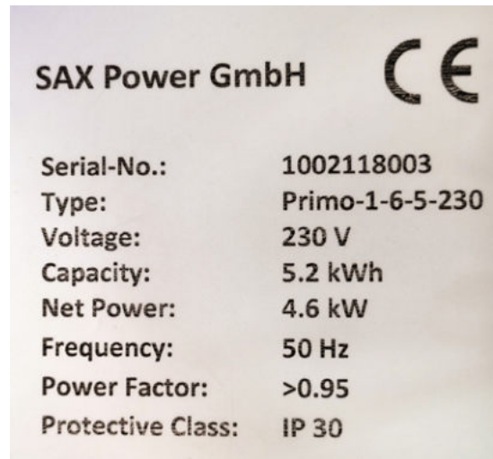
Typenschild des SAX-Homespeichers
